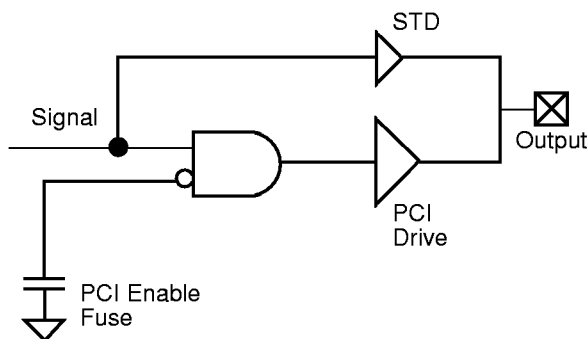
Figure 17 • I/O Module
